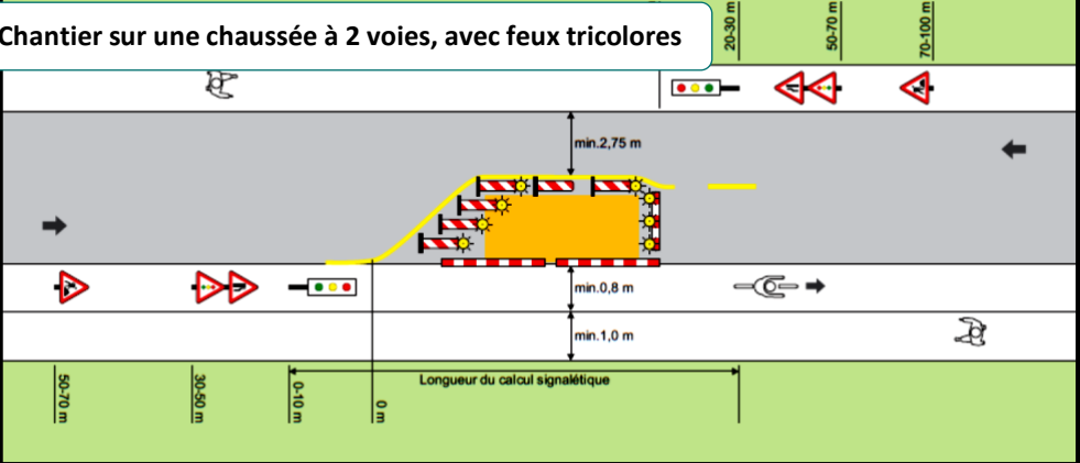
Chantier sur une chaussée à 2 voies, en milieu de chaussée
